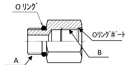
AU07(V)リングポート
