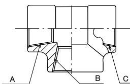
二面付きチーズ (210K/メッキ)
