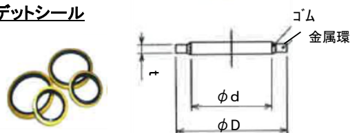
ボンデッドシール
